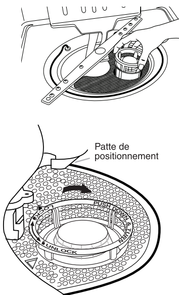
Réinstallation du filtre supérieur
